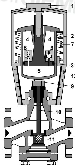
Szelep nyitva
