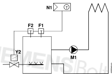
Szobatermosztát álló gázkazán közvetlen szabályozásával
