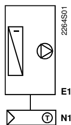
Szobatermosztát hűtő egység közvetlen szabályozásával
