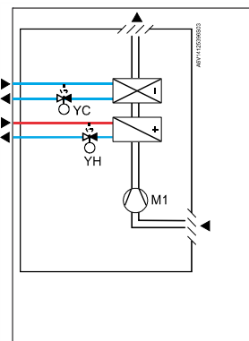
4-pipe fan coil unit
