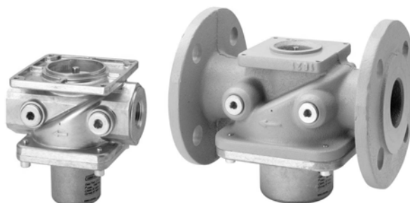
VGG...
