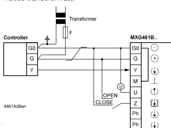
Közös transzformátor
