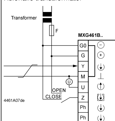
Különálló transzformátor
