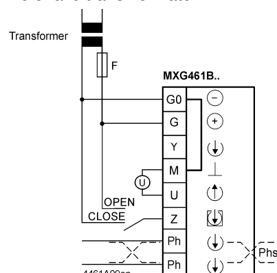
Különálló transzformátor
