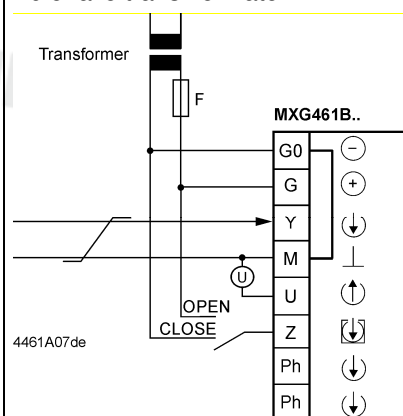
Különálló transzformátor
