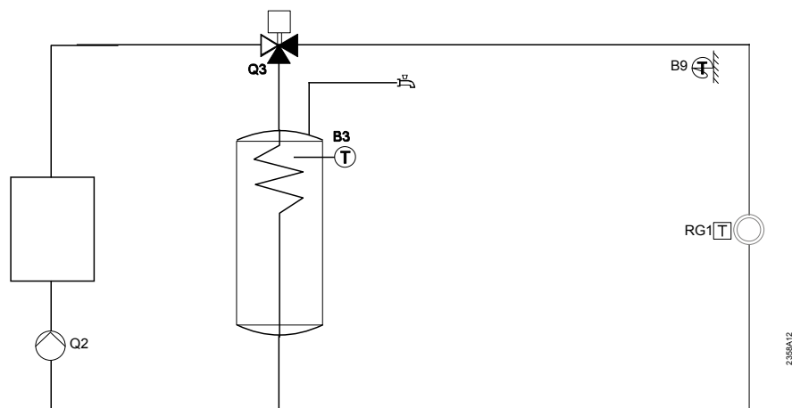
HMV fűtés váltószeleppel
