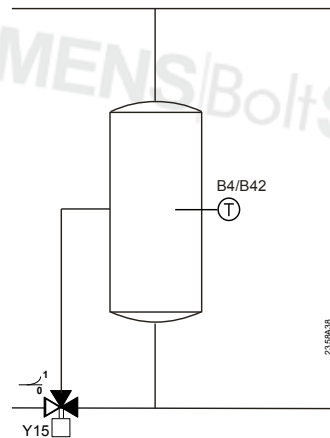
Puffer résztöltés
