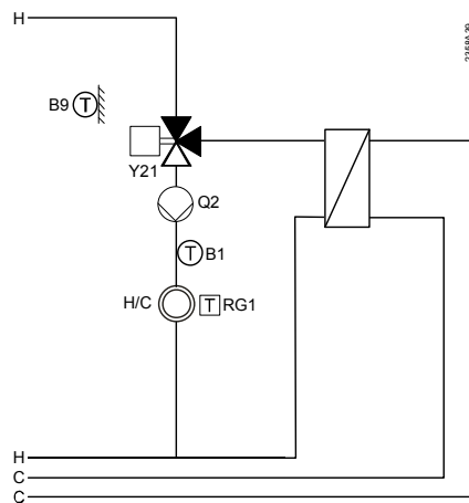
Hűtés váltószelep
