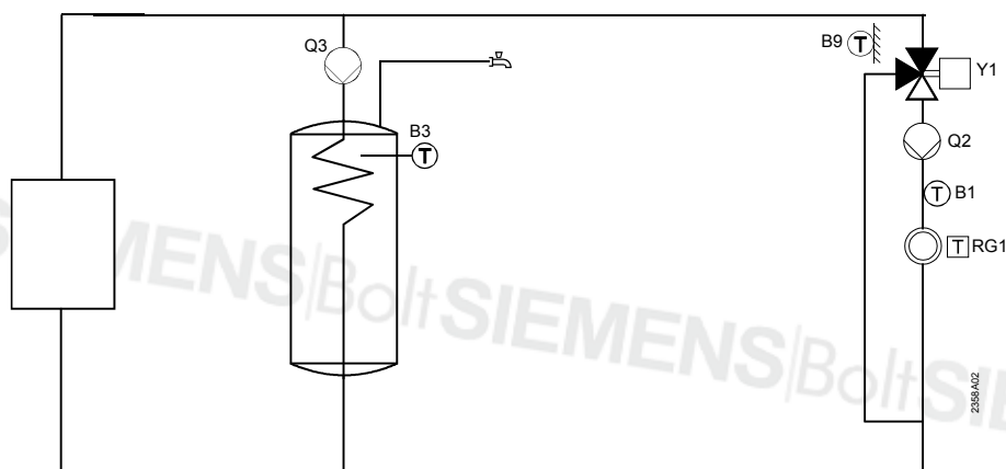
HMV fűtés váltószeleppel
