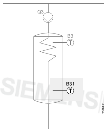
2. HMV érzékelő
